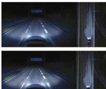
Tompított fényű fényszóró az autópályán (felül), javított látási viszonyok autópályafénykévével (alul)
