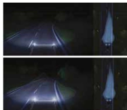
Tompított fényű fényszóró kedvezőtlen időjárási körülmények esetén (felül), javult látási viszonyok kedvezőtlen időjáráskor használatos fénykévével (alul)
