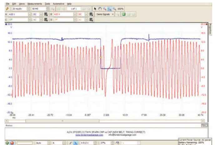
5. ábra: „utána” (új szíj, helyes beállítás)
