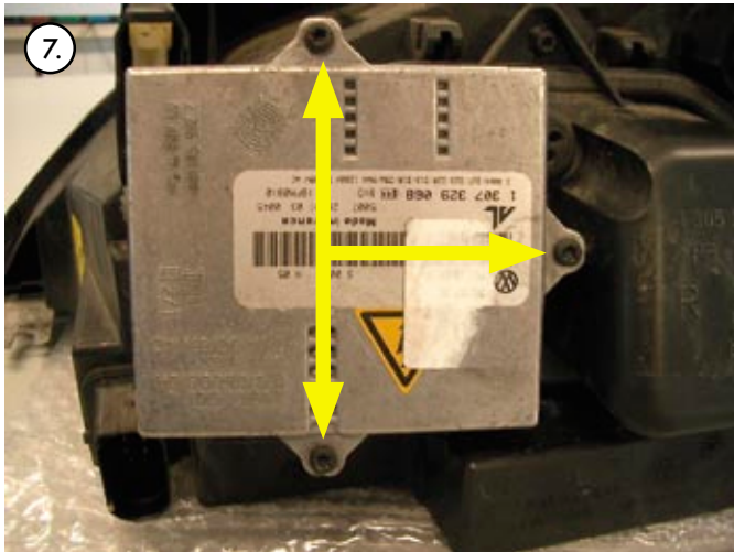
Az elektronikus egység rögzítőcsavarjait csavarozzuk ki!
