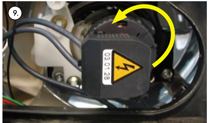
A gyújtóegységet ütközésig fordítsuk el balra, majd húzzuk le a xenonlámpáról!
