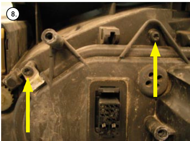
A fényszóróház borítását rögzítő csavarokat csavarozzuk ki!
