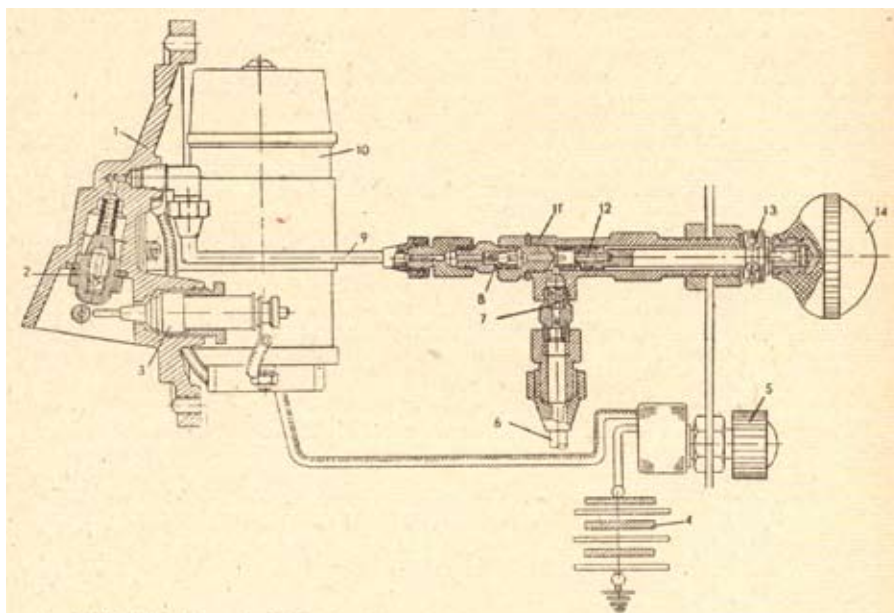
A JAAZ-200 típusú gépkocsi Diesel-motorjának indító-előmelegítő berendezése.
