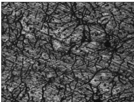
8 9 Az 1500 órát teljes terheléssel járatott motor kiindulási és kopott hengerfelületéről készített lenyomat képe
