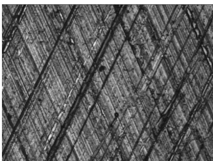
10 11 12 A spirálhónolt hengerfelület kiindulási, 40 és 140 órás kopott állapotáról készített lenyomat képe
