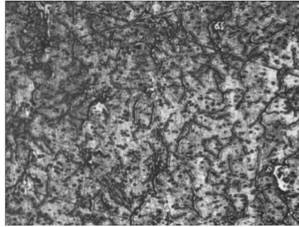
13 14 15 A lézerkezelt hengercsőfelület kiindulási, 40 és 140 órás kopott állapotáról készített lenyomat képe
