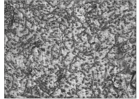
13 14 15 A lézerkezelt hengercsőfelület kiindulási, 40 és 140 órás kopott állapotáról készített lenyomat képe
