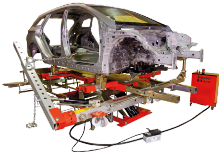
6 A B15 Supert felszerelték elektromos működtetésű hidraulikával
