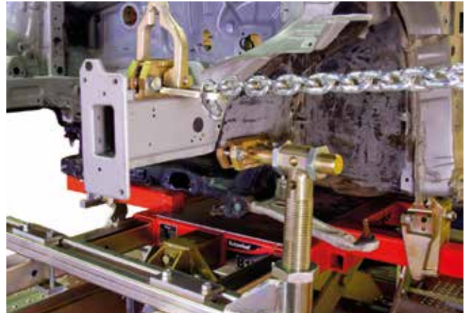
9 Zártszelvény egyengetése támasztó rendszerrel
