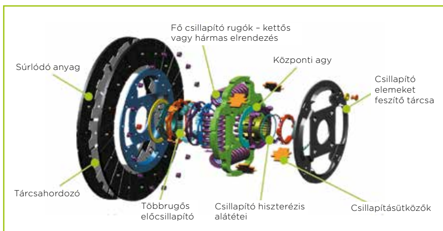
A Kit 4P kuplungtárcsája hosszú utas torziós csillapítóval van ellátva (Long Travel Damper)
